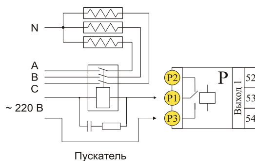
Рис 5.2 Типовые схемы подключения исполнительных устройств к релейным выходам.
