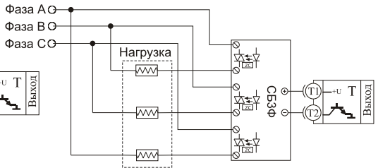
Подключение трехфазной нагрузки по шестипроводной схеме
