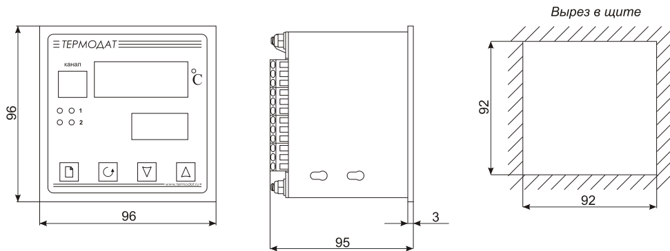
Основной блок
