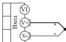
термопара
