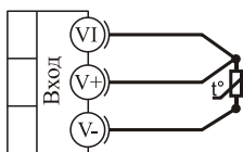
термометр сопротивления
