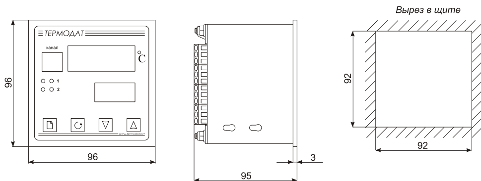
Основной блок
