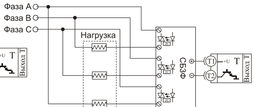
Подключение трехфазной нагрузки по шестипроводной схеме
