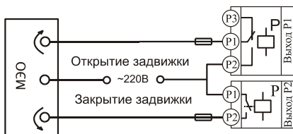
Подключение электрозадвижки
