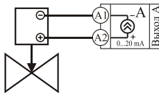
Подключение задвижки с электроприводом
