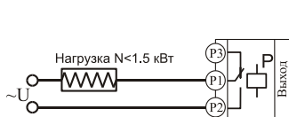
Подключение нагрузки менее 1,5 кВт
