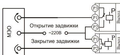
Подключение электродвиги
