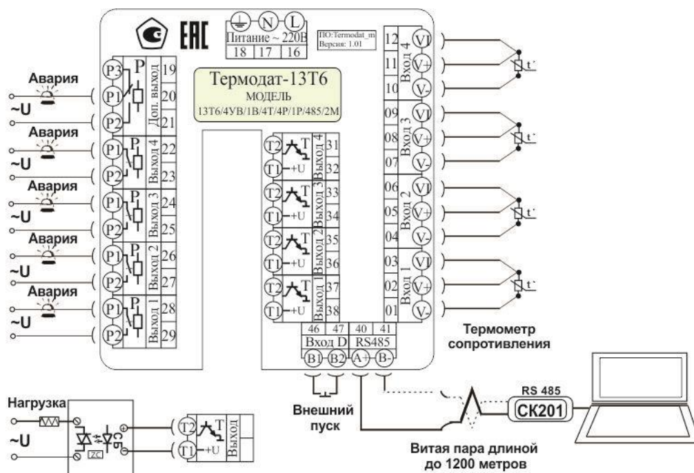
Рисунок 8. Схема подключения прибора.
