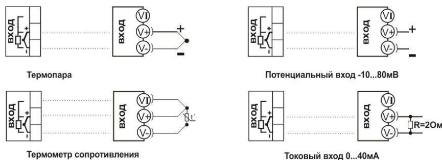
Рисунок 5. Схемы подключения датчиков.
