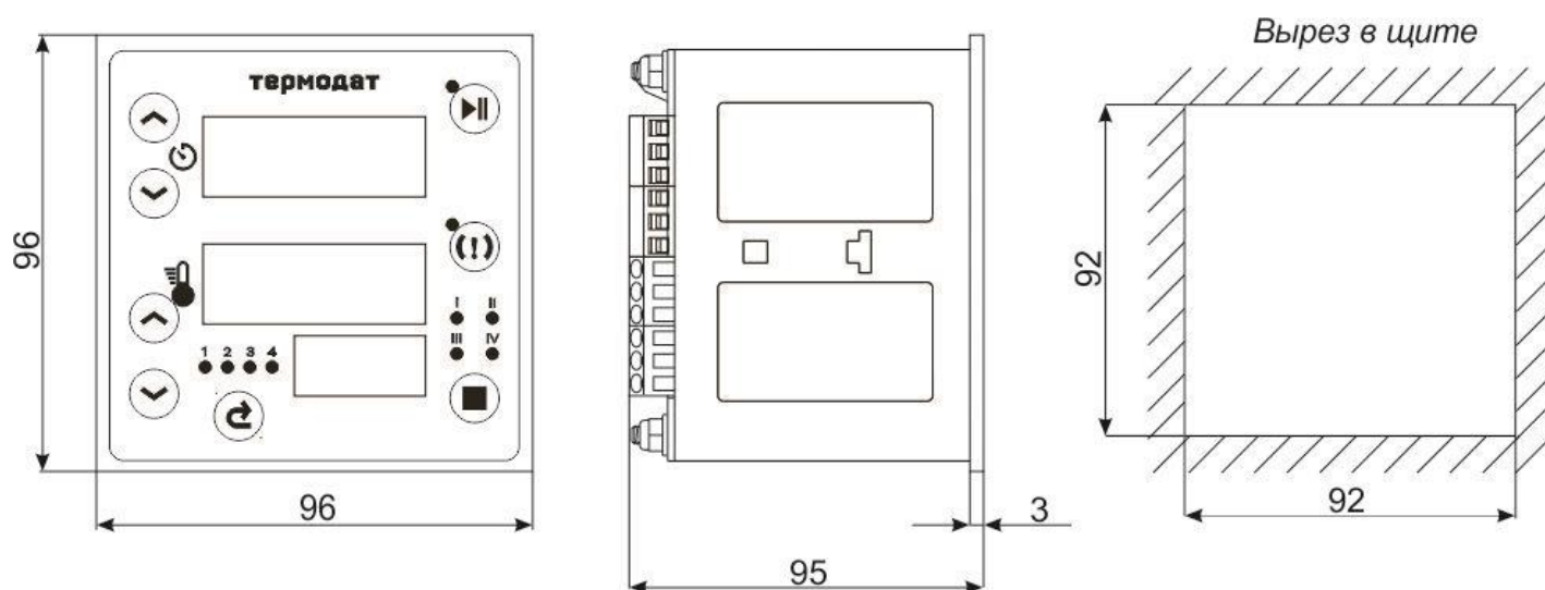
Рисунок 9. Габаритные размеры прибора Термодат-12Т6/...
