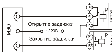
Подключение электрозадвижки
