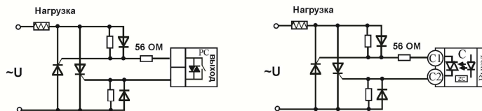
Подключение внешних тириستоров
