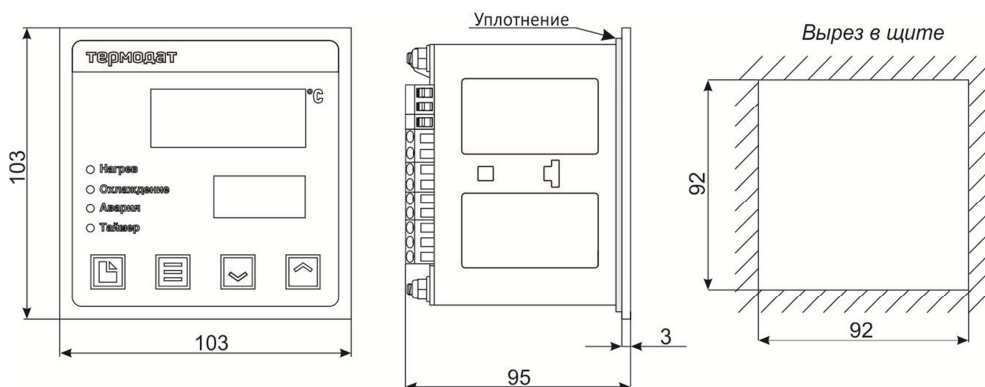
Рисунок 18 – Габаритные размеры прибора Термодат-12К6-D4/...../ IP67пп
