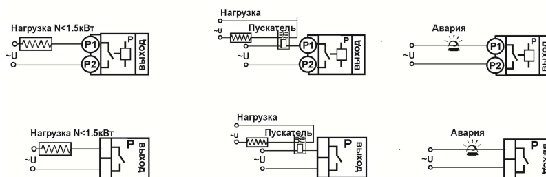
Подключение нагрузки менее 1,5 кВт
