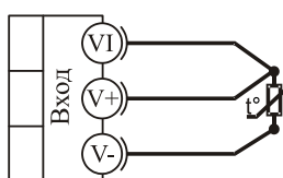
термометр сопротивления
