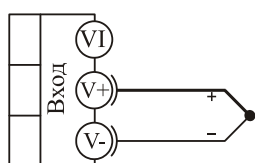
термопара
