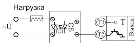
Управление однофазной нагрузкой с помощью блока СБ
