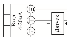
датчик с унифицированным токовым сигналом и питанием от прибора
