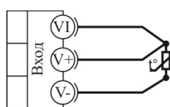
термометр сопротивления
