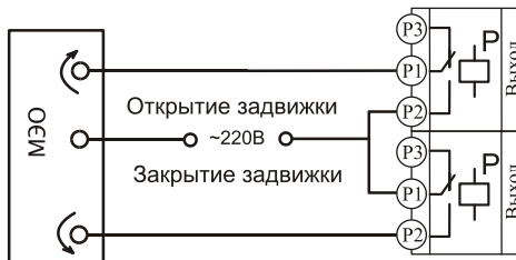
Подключение электрозаводки
