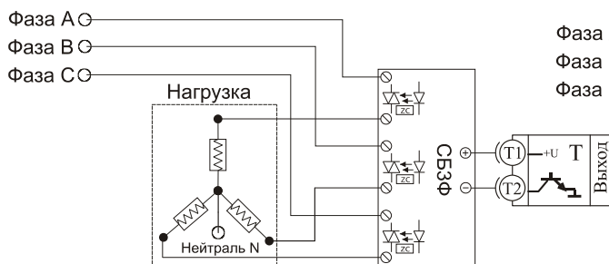
Управление трёхфазной нагрузкой с помощью трёхфазных силовых блоков. Схема подключения "Звезда с нейтралью"
