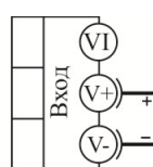
0...80 мВ потенциальный вход
