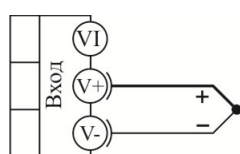
термопара
