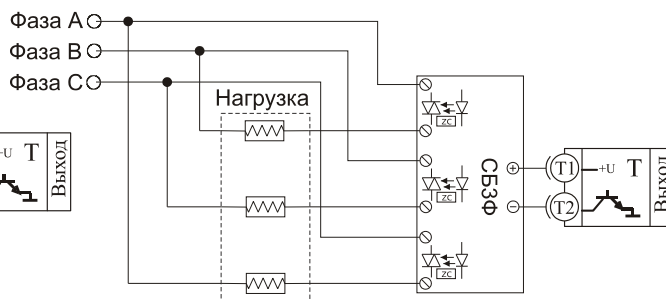
Подключение трёхфазной нагрузки по шестипроводной схеме
