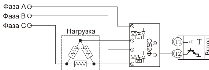
Использование двухфазных силовых блоков для управления трёхфазной нагрузкой. Схема подключения "Треугольник"
