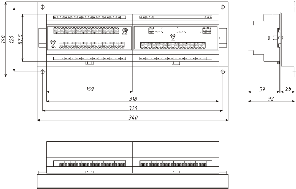
Периферийный блок
