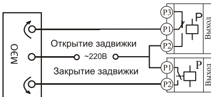
Подключение электрозадвижки
